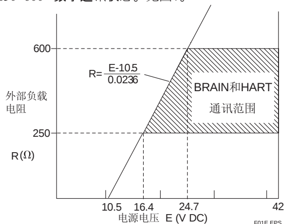
图1 电源电压与负载电阻关系
